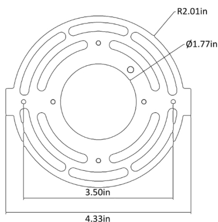
Gabarit de perçage pour montage en saillie
