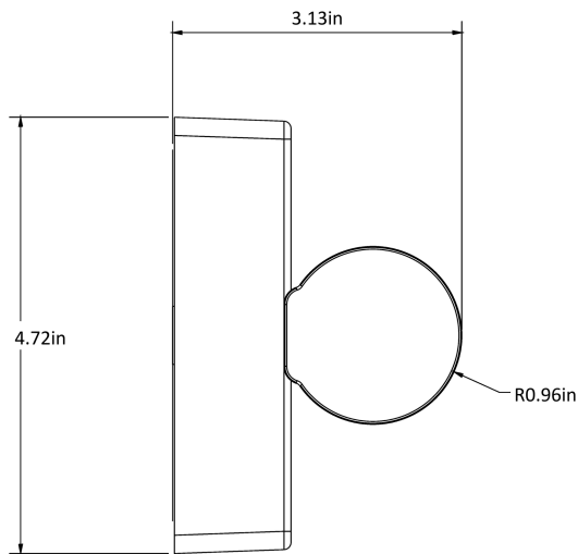
CS-CY-02-22W Side View
