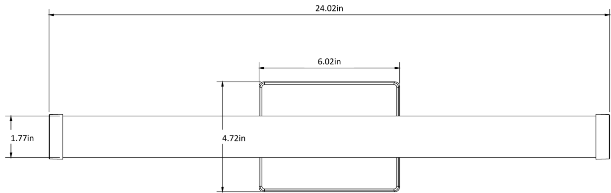
CS-CY-02-22W Front View · 24.02in long · 6.02in canopy · Ø1.77in tube
