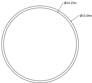
CS-EC-15-24W Front View
