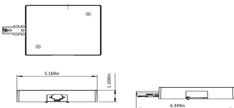
H10021 Alim. d'extrémité, circuit unique
