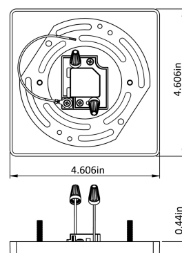
H10016 Adaptateur monopoint
