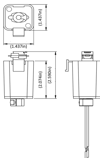
H10011 Adaptateur de luminaire suspendu à cordon
