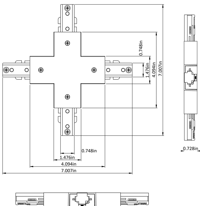
H10004 Connecteur en X
