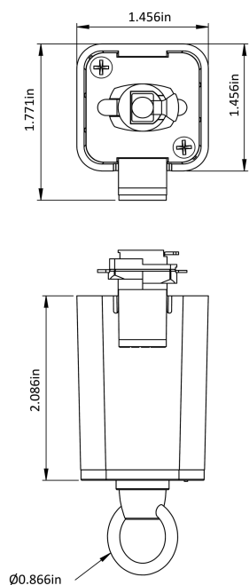
H10010 Adaptateur de luminaire suspendu à chaîne
