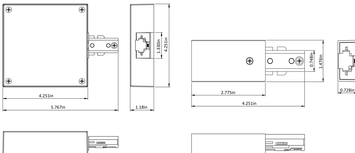
H10013 Alim. d'extrémité pour barre en T
