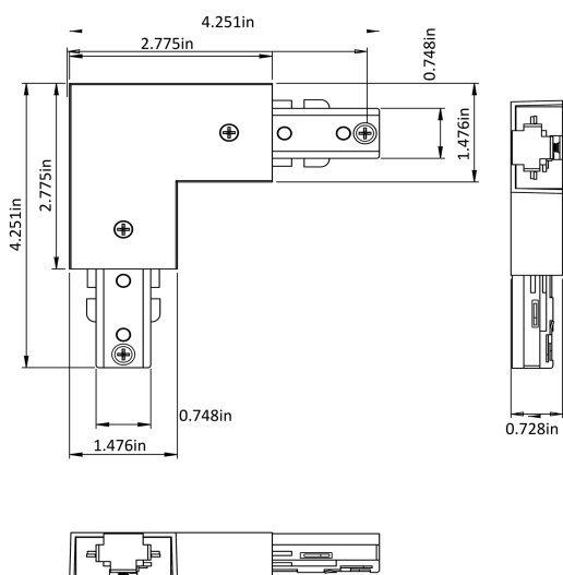
H10003 Connecteur en L
