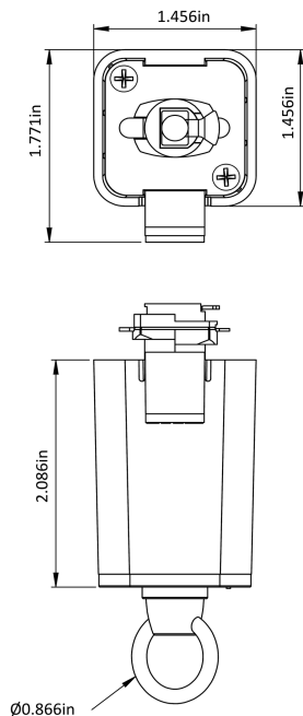
H10010 Pendant luminaire adapter chain
