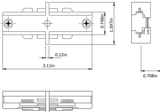
H10001 Mini connector
