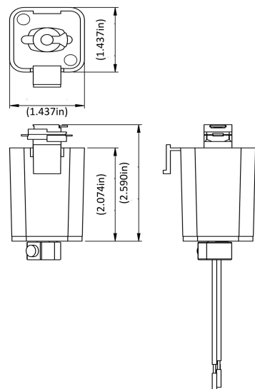
H10011 Pendant luminaire adapter cord
